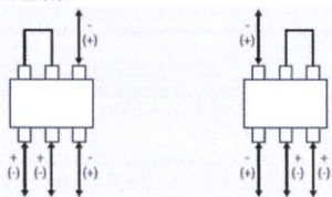
接线方式1
